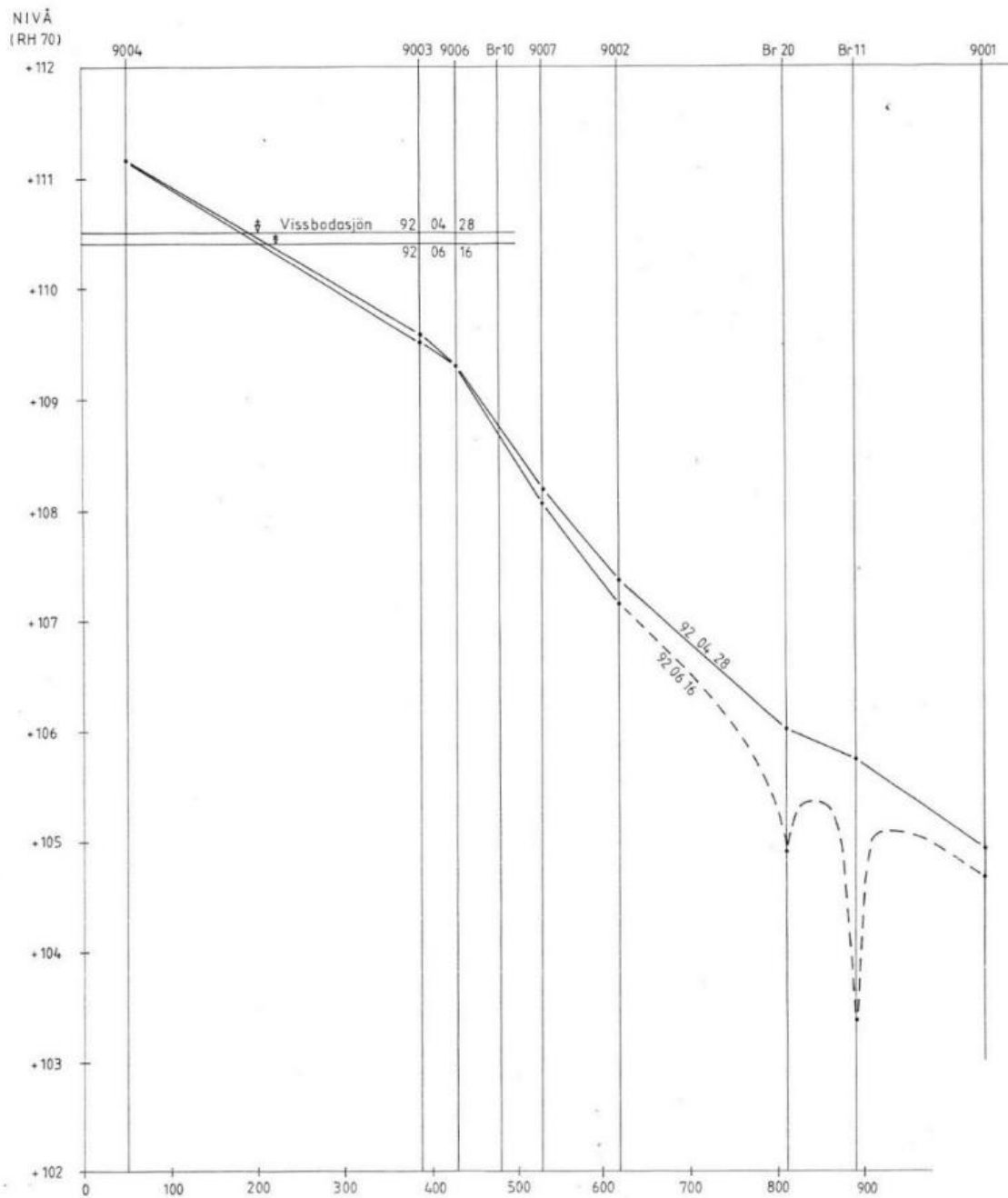
Figur 3.5. Profil med grundvattennivåer vid ostörda förhållanden (inget uttag, ingen infiltration) samt efter sex veckors försök med grundvattenuttag i Br11 (8,3 l/s), återinfiltration (8,3 l/s) samt grundvattenuttag i Br20 (11 l/s). Från VBB Viak, 1995.
