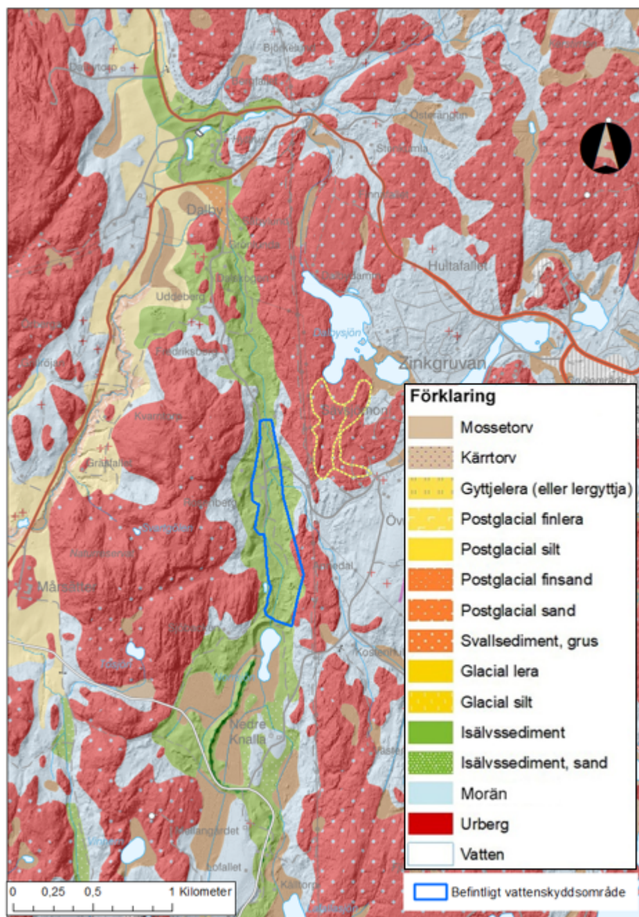
Figur 3.2. Jordartskarta över Forsåsens (©SGU) med läge för befintligt vattenskyddsområde.
